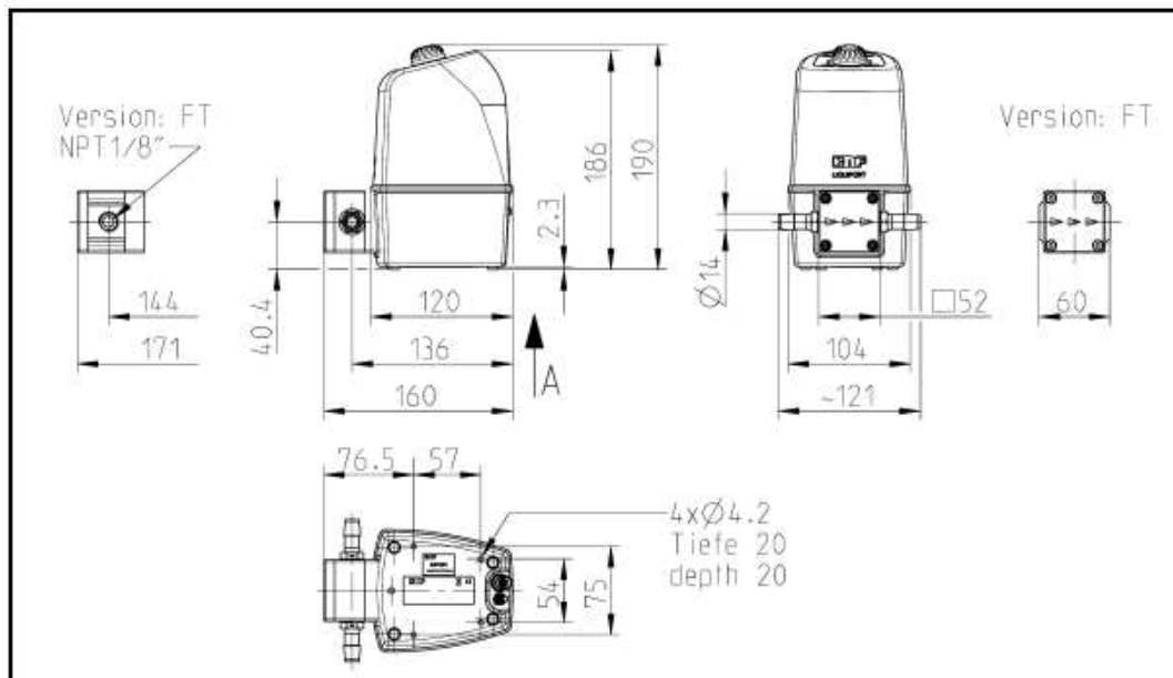
Fig. 3: Mounting dimensions LIQUIPORT 300 / LIQUIPORT 1.300
