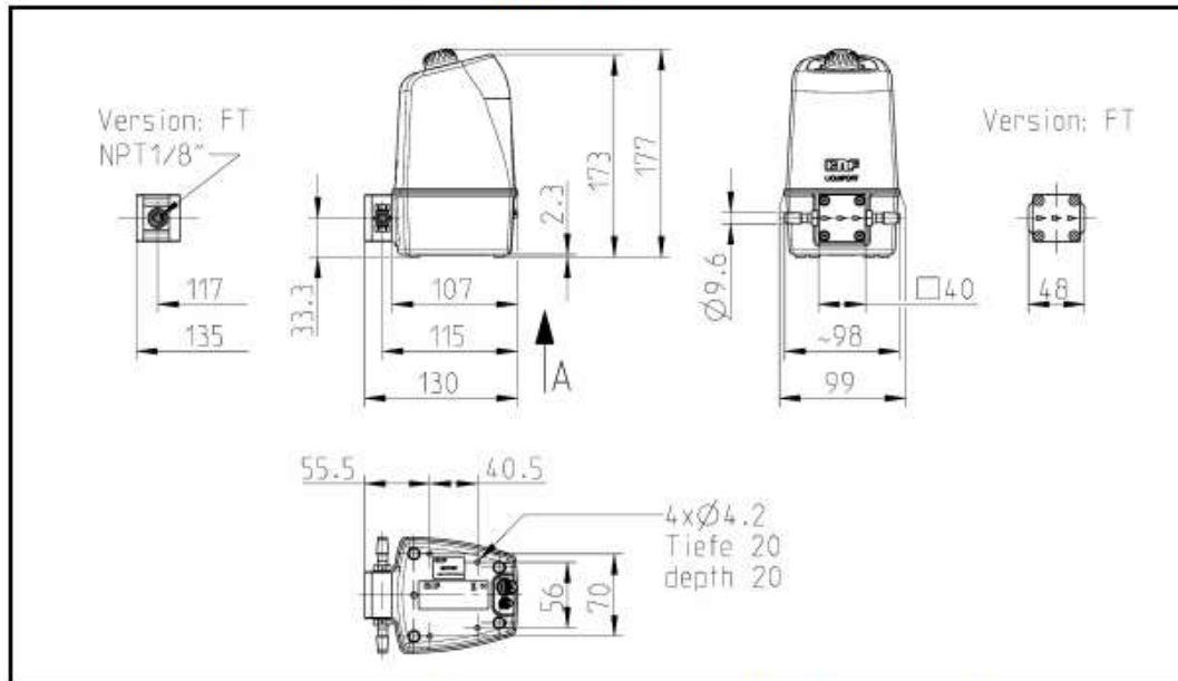
Fig. 2: Mounting dimensions LIQUIPORT 100 / LIQUIPORT 1.100
