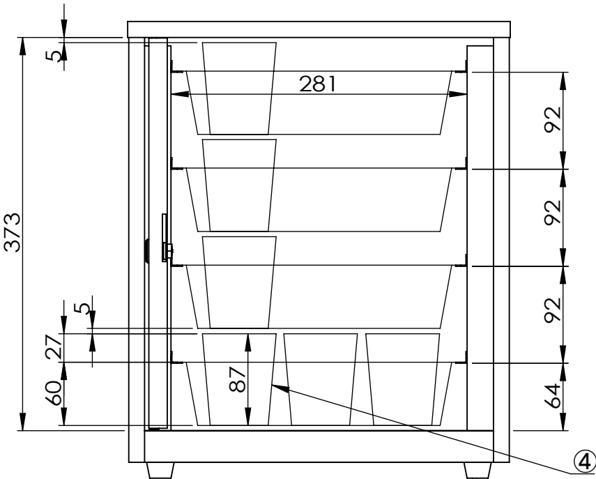
扉開口時
