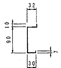
A A 断面図
