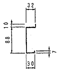
B B 断面図
