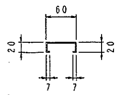
C C 断面図
