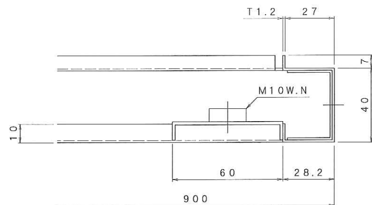
A部 詳細図 (S=1/2)
