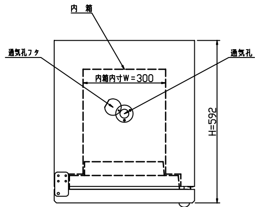
平面図
