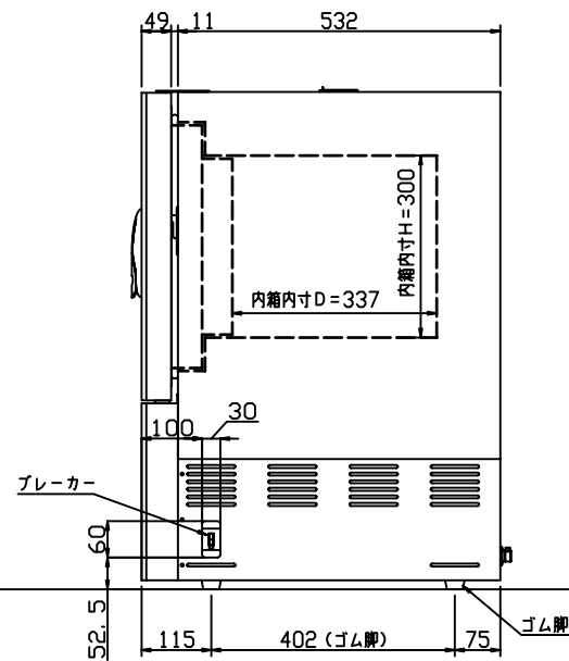
右側面図
